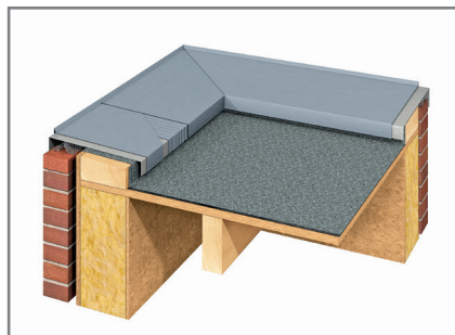
Raccord de couvertines en toiture-terrasse
