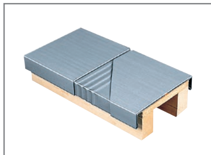
Sección en detalle de revestimiento de peto
